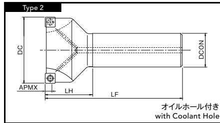
オイルホール付き with Coolant Hole
