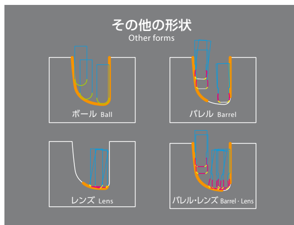
加工範囲 Machined area
