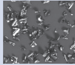
スレッドミルの切りくず Chips from thread mill
