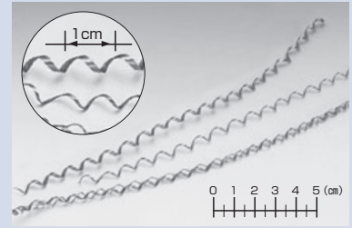
スパイラルタップの切りくず Chip from a spiral fluted tap
